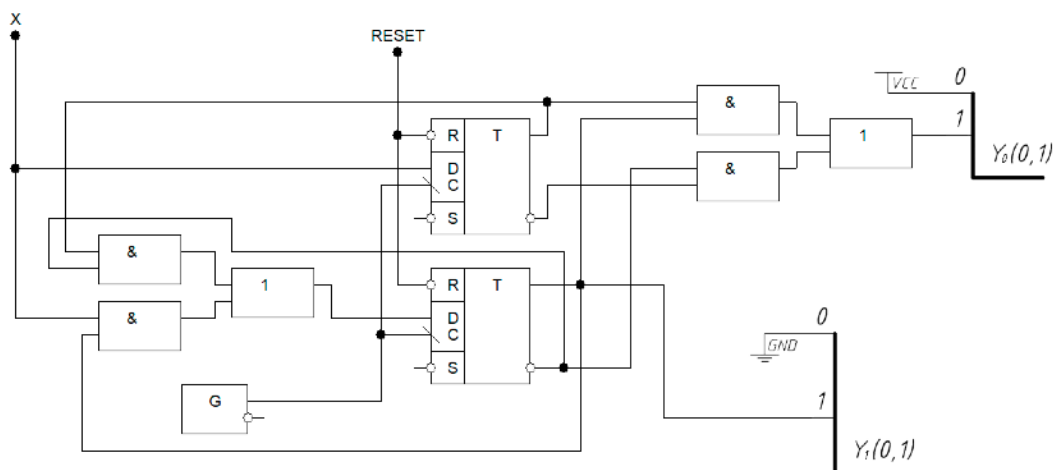
Рисунок 9 – Итоговая логическая схема автомата Мура
