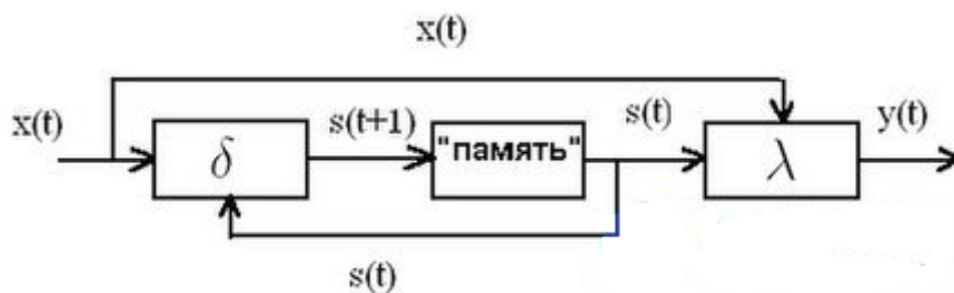
Рисунок 5 – Обобщенная структурная схема автомата Мили
