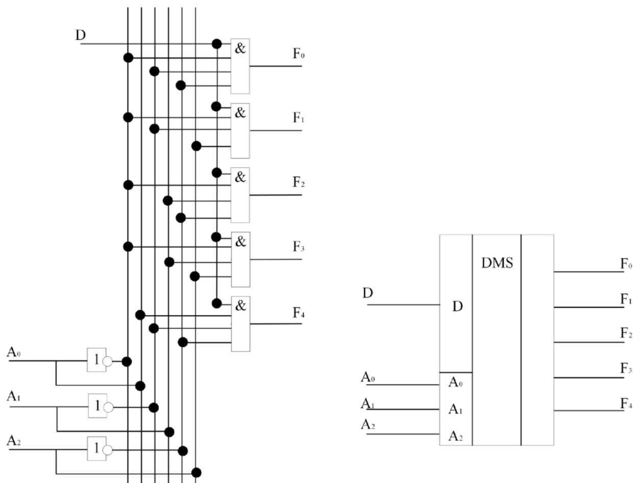
Рисунок 2 - Структура и УГО демультиплексора «из 1 в 5»
